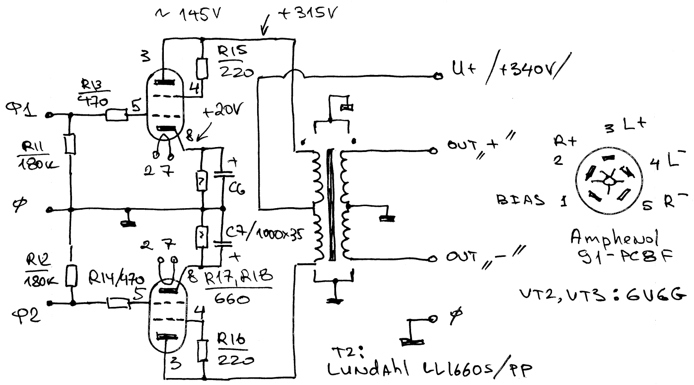
Рис 2. ВЫХОДНОЙ КАСКАД
