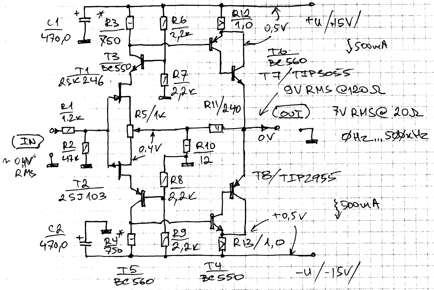
①. Усилитель
